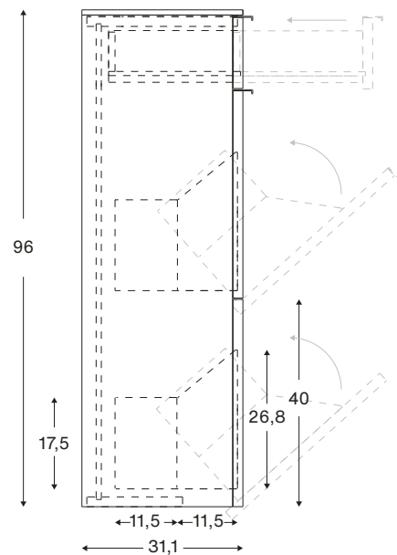
Zweireihige Schütte / Double-row bin
