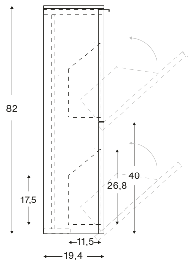
Einreihige Schütte / Single-row bin
